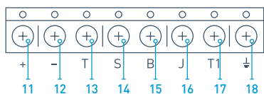
Рис. 18. Служебные выходы приемника осBridge и клеммы питания
