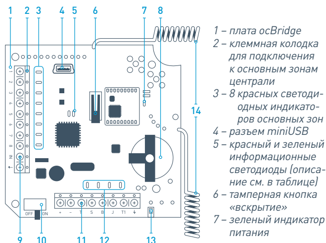
РИС. 1. Приемник беспроводных датчиков ocBridge
