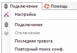
РИС. 9 Меню «Подключение»
